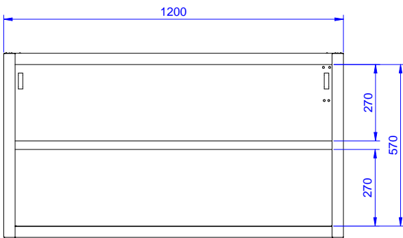
Front aanzicht
